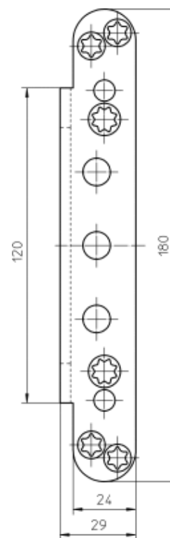
вид спереди
